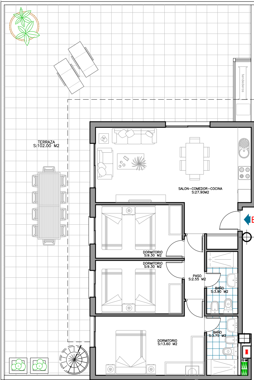
PLANTA ATICO
